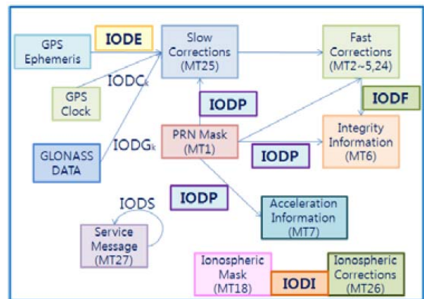
Fig. 2. SBAS message flow chart (RTCA 2001).
