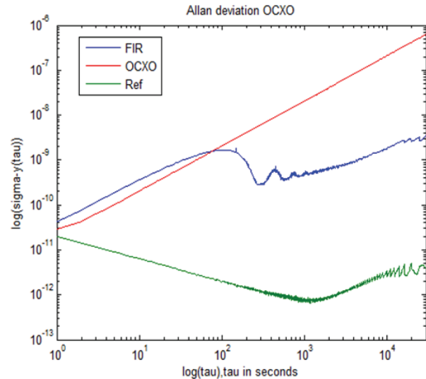
(b) OCXO
